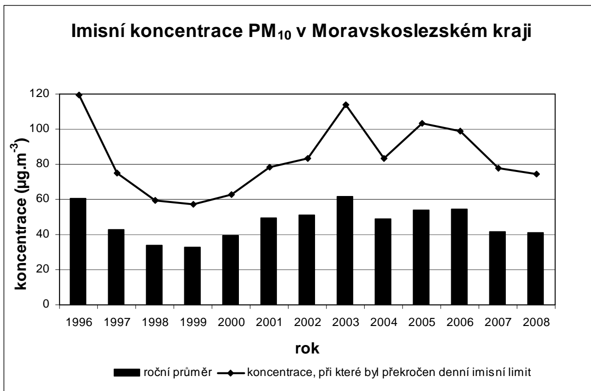
Obr. 1 Vývoj imisních koncentrací suspendovaných částic PM 10 v Moravskoslezském kraji za roky 1996 – 2008 (zdroj ČHMÚ) 1 .
